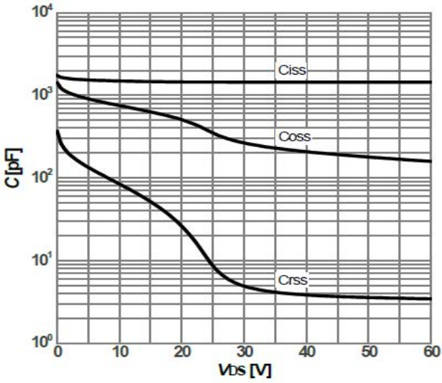
Typ. capacitances
